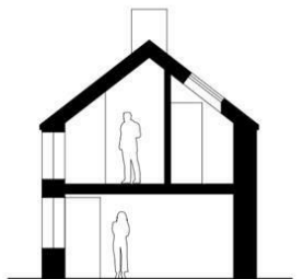
7 Section A-A Scale: 1:100
